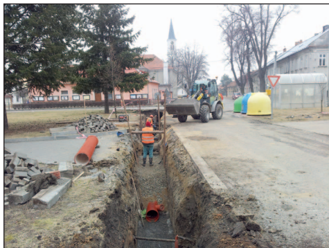
Začátkem března zahájili pracovníci Sdružení INSTA CZ-STRABAG výstavbu prvního úseku kanalizace, na kterou obec získala dotaci.
